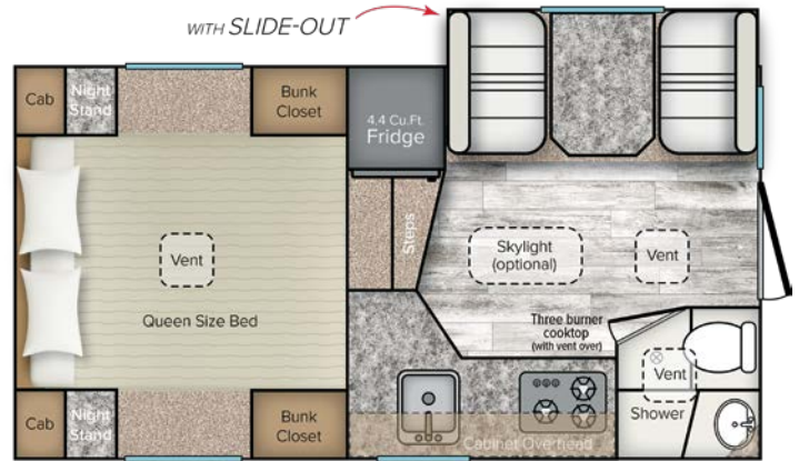
TRAVELAIRE 8.3 SL
