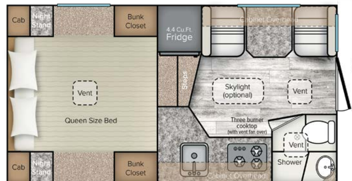
TRAVELAIRE 8.0 WS
